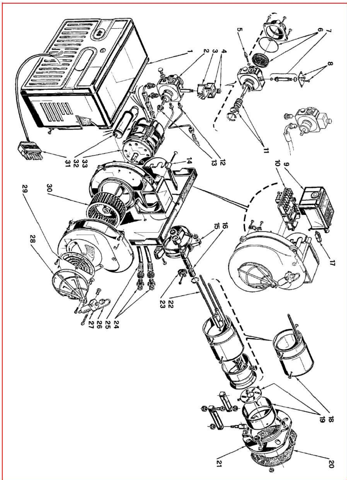
RIELLO 40 G10 COD. 3746412 - 3746414 Bruciatori di gasolio • Light oil burners • Brûleurs fioul • Öl-Gebliäsebrenner Quemadores de gasóleo TIPO / TYPE / TYP 464 T1
